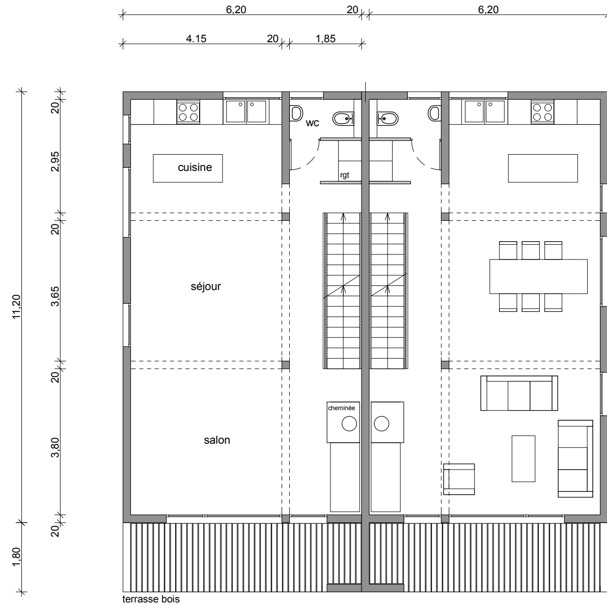
REZ-DE-CHAUSSEE surface SHON : 62,30 m 2
